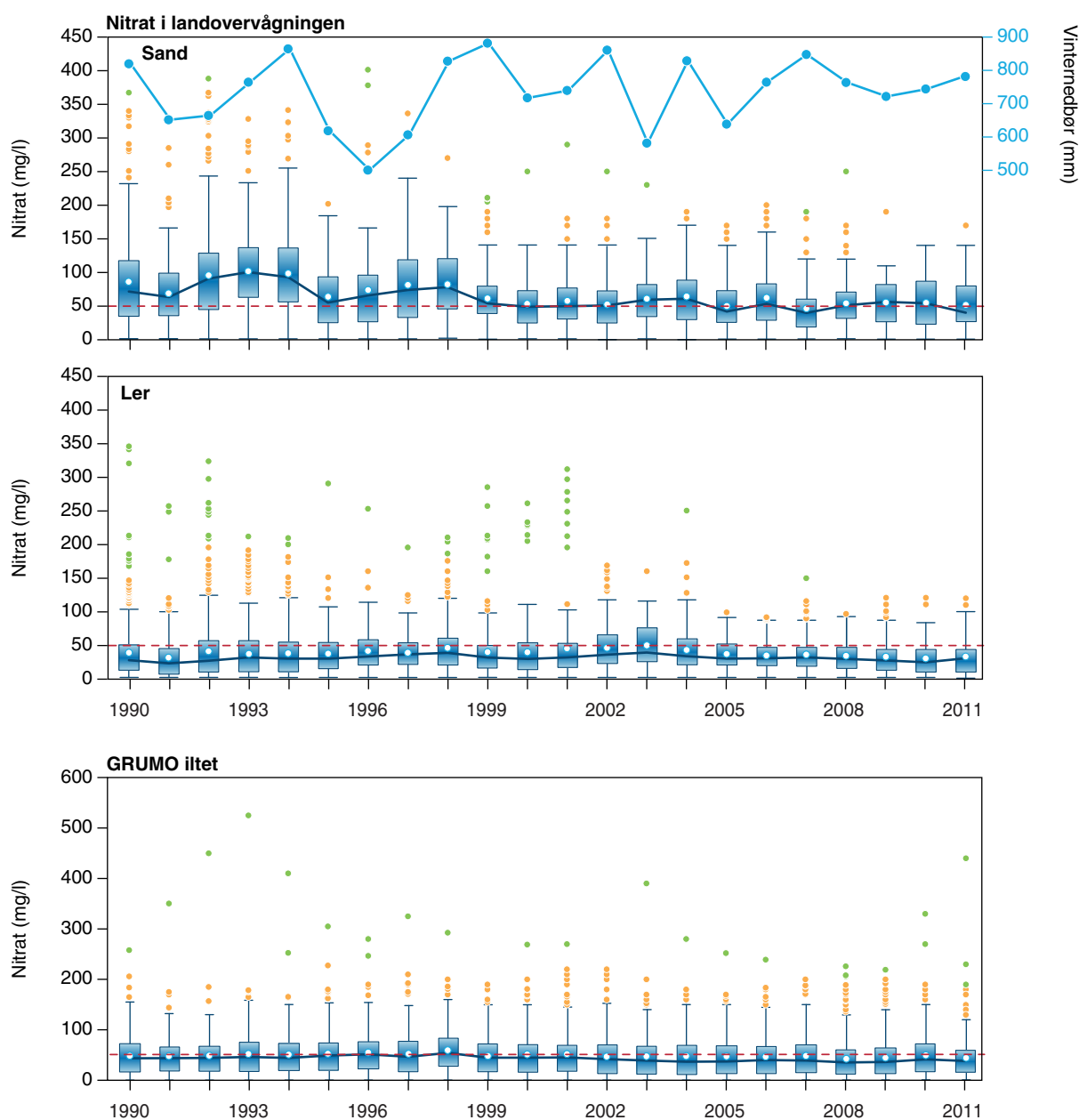
Figur 6.5. Udviklingen i nitratindehold i grundvand i perioden 1990-2011. Øverst er vist resultater fra landovervågningsområders højtliggende grundvand i sand- og lerjordsområder sammenlignet med vinternedbøren (øverste kurve). Kun nitratanalyser >1 mg/l og indtag ned til 6 m's dybde. Nederst er vist resultater fra det iltede grundvand i grundvandsovervågningsområderne. Kurven i boksen forbinder medianværdierne. Desuden er vist 75 % og 25 % fraktiler i minimums og maksimumsværdier af analyseresultater det enkelte år, samt grænseværdien for nitrat i drikkevand og grundvand på 50 mg/l. Grønne prikker viser målinger større end 75 % fraktil + 3(75 % fraktil - 25 % fraktil). Orange prikker viser større end 75 % fraktil + 1,5(75 % fraktil - 25 % fraktil) (Thorling et al. 2012).
