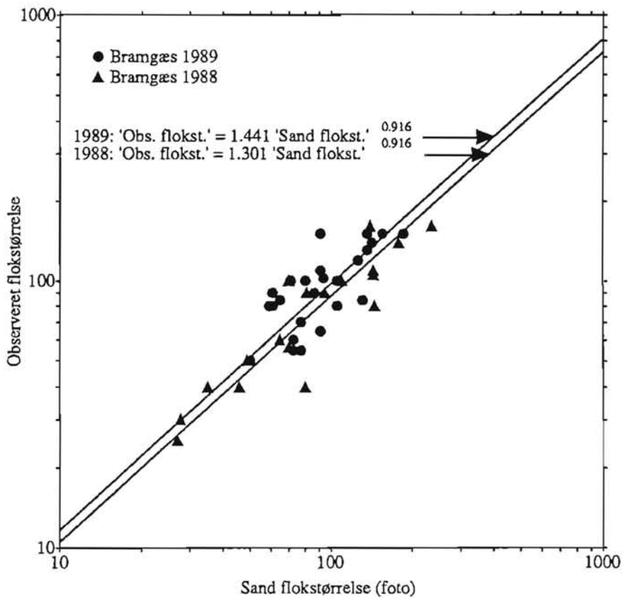
Figur 5.3 Observerede flokstørrelser versus sande flokstørrelser af Bramgæs i 1988 og 1989 i logaritmsk plot.
