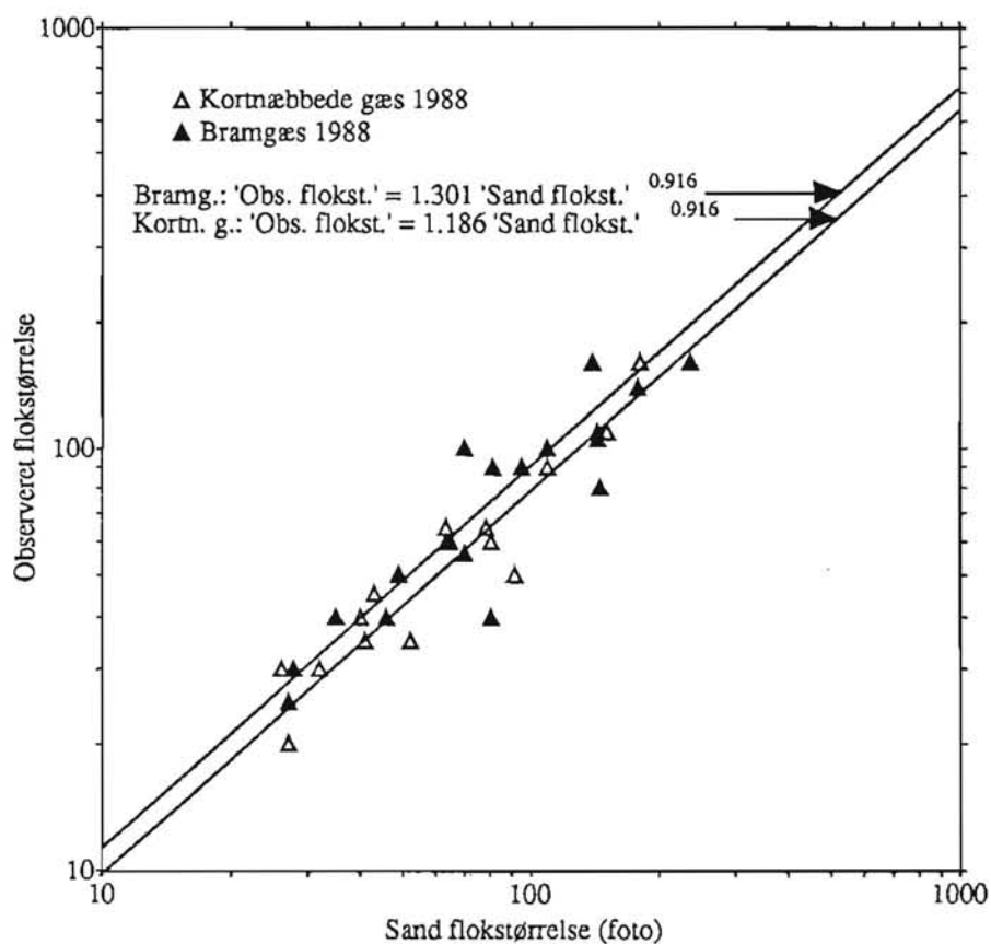
Figur 5.5 Observerede flokstørrelser versus sande flokstørrelser af Kortnæbbede Gæs og Bramgæs i 1988 i logaritmsk plot
