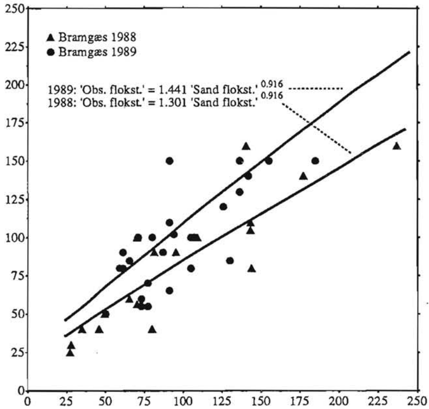
Figur 5.2 Observerede flokstørrelser versus sande flokstørrelser af Bramgæs i 1988 og 1989 i ikke-logaritmsk plot.
