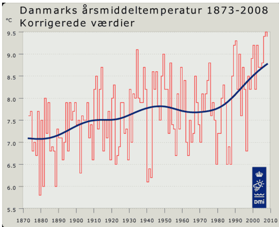
1 2 Figur 2.3: Danmarks årsmiddeltemperaturer 1873-2008. Kilde: DMI 2009c
