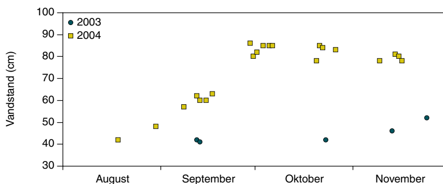
Figur 13. Vandstand i Vesterenge i perioden august-november 2003 og 2004. Vandstanden blev aflæst på en vandstandspæl. Vandstandspælen blev flyttet fra 2003 til 2004, og værdierne er derfor ikke sammenlignelige imellem de to år.
